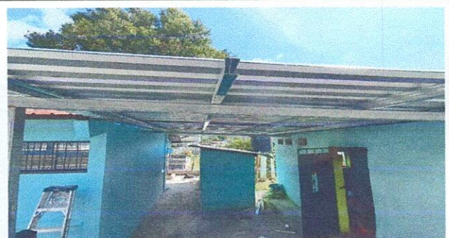
Foto 4: Mejoramiento de techo de cocina y aula.
